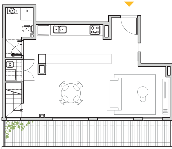
1° NIVEL
