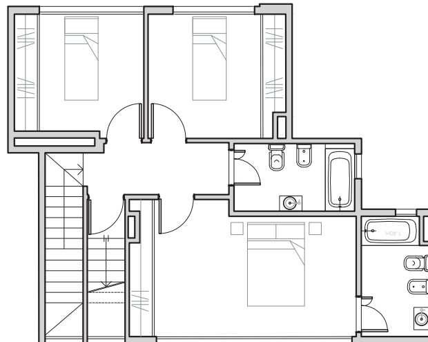
2° NIVEL
