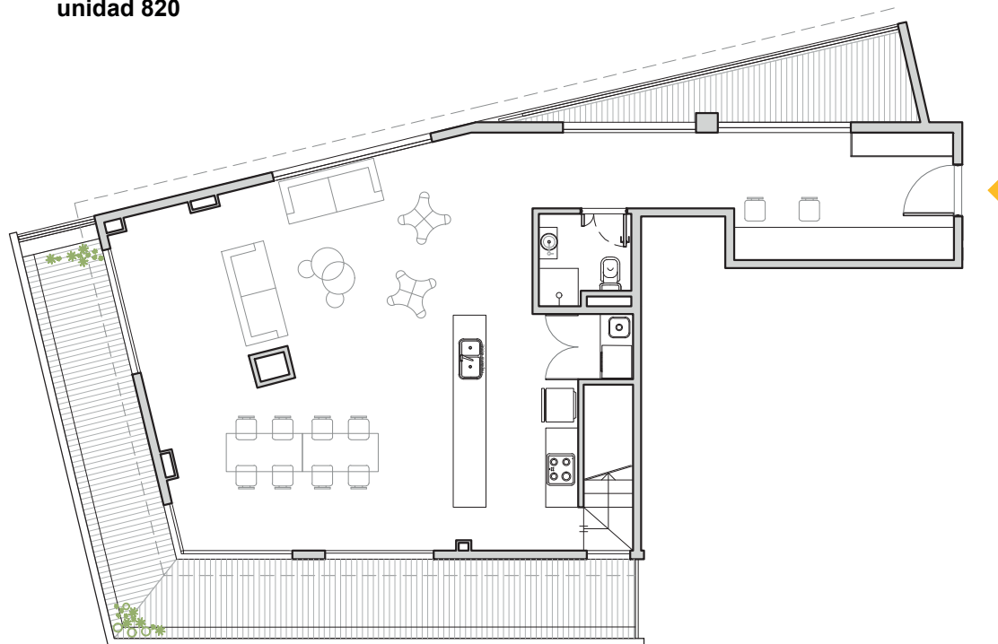
1° NIVEL
